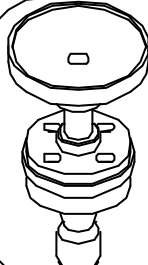
IPH-4541 PICK-UP NOZZLE \phi 20 -LL (OD= \phi 20.0 ) FUJI, IP2
