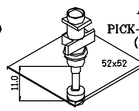
AQNA-3258 PICK-UP NOZZLE \phi 7.0 (OD= \phi 7.0 ) FUJI , IP3
