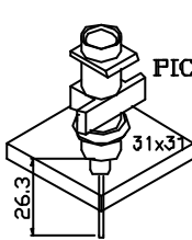
AQNA-3340 PICK-UP NOZZLE \phi 1.3 (OD= \phi 1.3 ) FUJI , IP3
